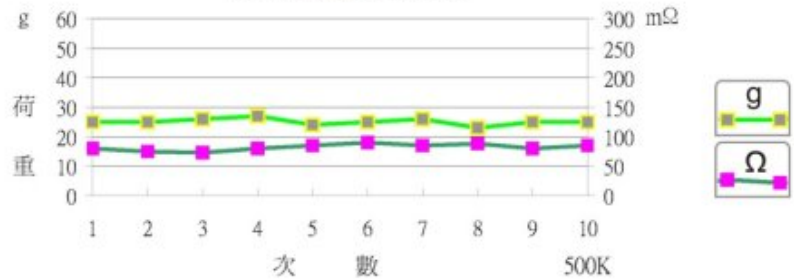
荷重阻抗試驗曲線圖
